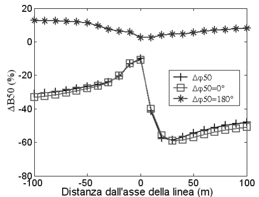
Figura 4. Errore percentuale sul livello di esposizione mediano, \Delta B_{50} , dovuto all'Eq. (36) con \Delta\phi_{50} (valore centrale della serie di valori di \Delta\phi ), \Delta\phi_{50} = 0^\circ , \Delta\phi_{50} = 180^\circ , per la linea di Fig. 1 (carico giornaliero di Fig. 2). Altezza dal suolo 1 m.
